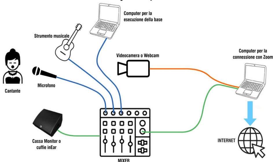
Schema di collegamento per le audizioni on line
